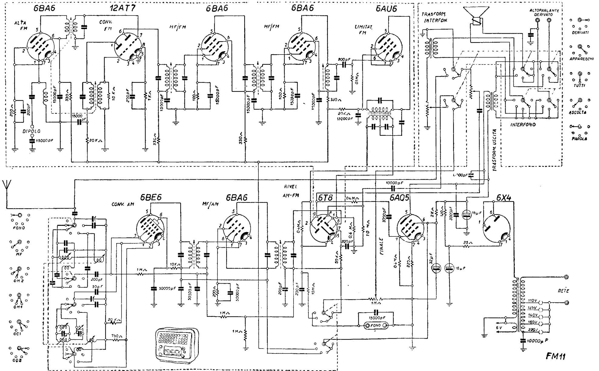
REOM - Sintomagic Radio mod. FM11 - Apparecchio a modulazione d'ampiezza e di frequenza, con dispositivo multivox. Consente conversazioni bilaterali a viva voce e diffusione in altro ambiente dei programmi radio. Medie frequenze a 470 kc ed a 10,5 Mc. Rivelazioni AM e FM ottenuta con valvola 6T8.
